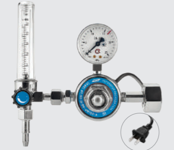
У-30/AP-40-P-01-1P (220V) арт. 001.010.610
