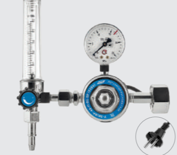
У-30/AP-40-P-01-1P (220V) арт. 001.010.611
