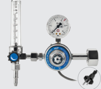
У-30/AP-40-P-1P (220V) арт. 001.010.601
