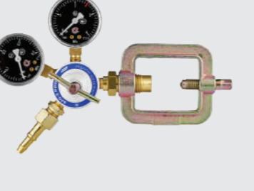
БАО-5 МИНИ арт. 001.010.302
