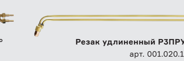
Резак удлиненный Р3ПУ, L=800, ∠150° арт. 001.020.163
