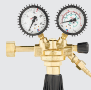
У-30/AP-40-КР-И арт. 001.010.605
